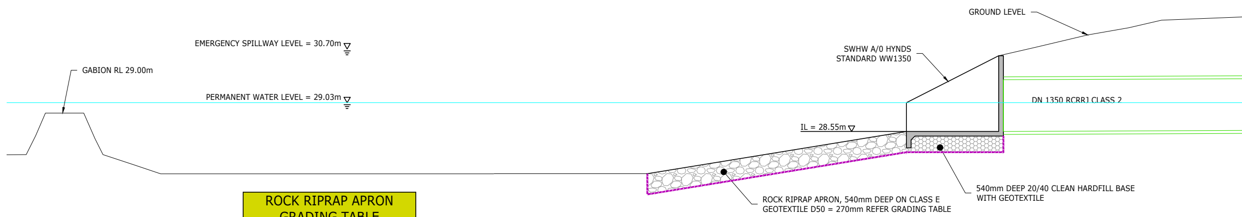
A STORMWATER OUTLET A/0 - A/1 SCALE 1:50 - A1, 1:100 - A3
